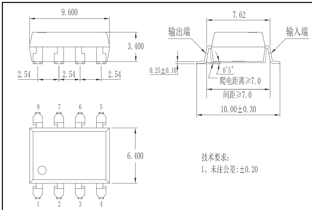
图 4 HSSR-DA09-2 外形尺寸
