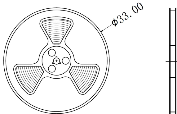
图 6 编带包装示意图 Figure 6- Taping Packing Schematic
