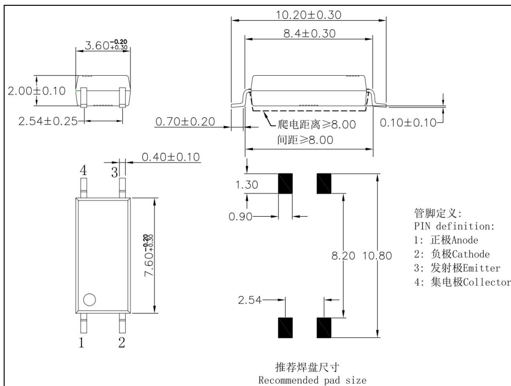
图 3 HPC101× 外形尺寸 Figure 3- The dimensions of HPC101×
