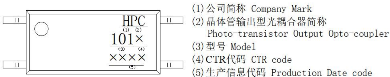
图 4 产品印章 Figure 4- Marking
